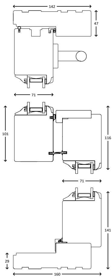
Vandret snit
