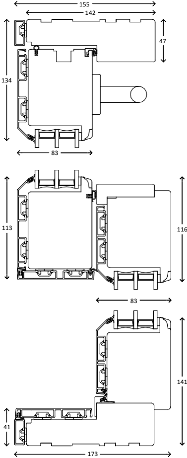
Vandret snit
