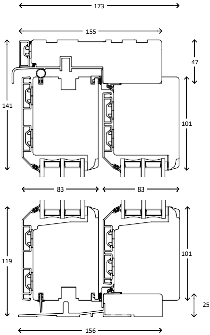
Lodret snit
